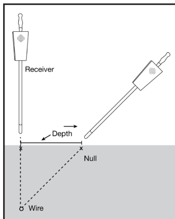
FIGURA 5: Determinación de la profundidad
