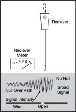
FIGURA 3: Localización del extremo de un cable roto
