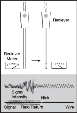
FIGURA 4: Localización de una melladura del cable
